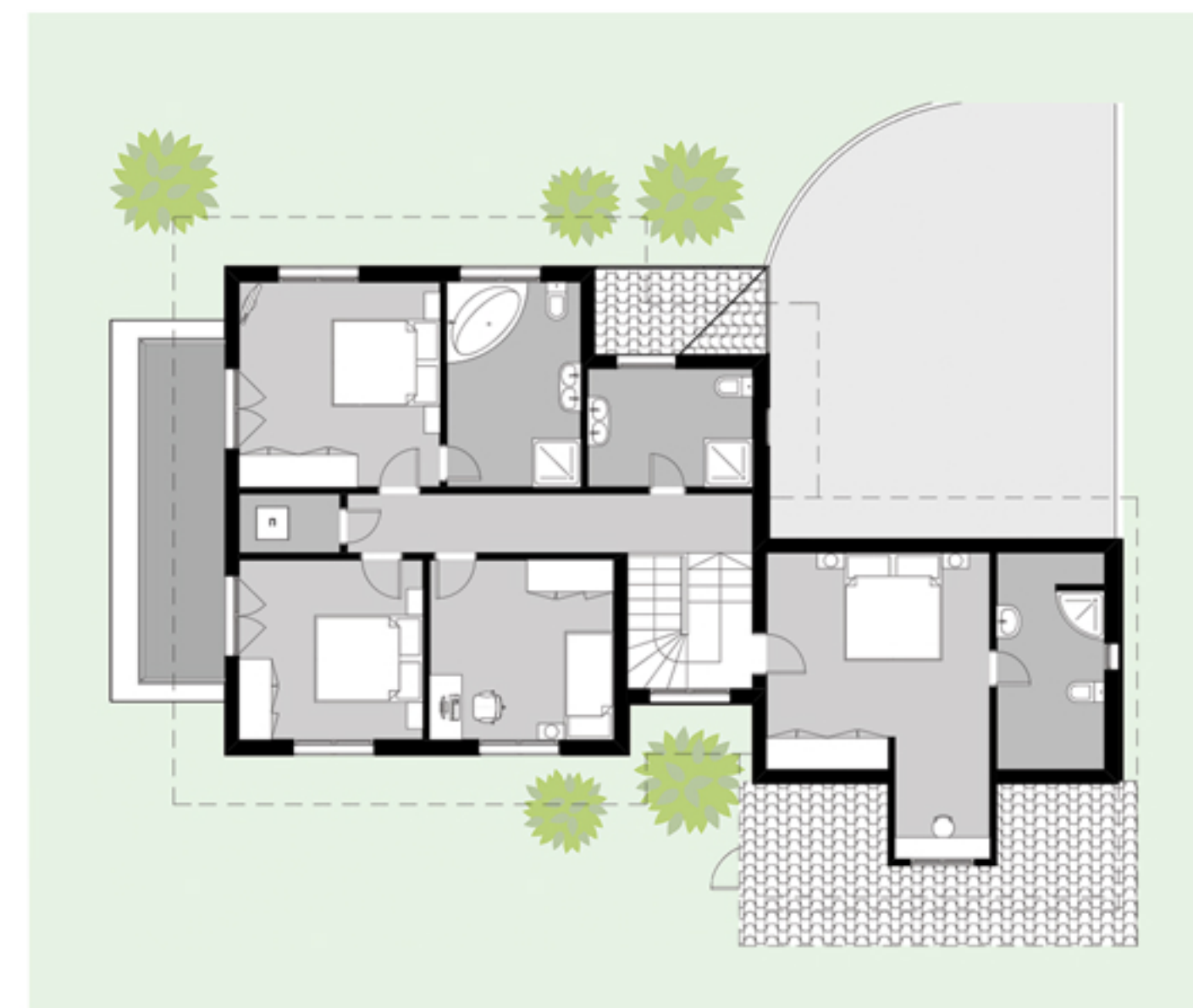
АРХИТЕКТУРЕН ПЛАН ВТОРИ ЕТАЖ
